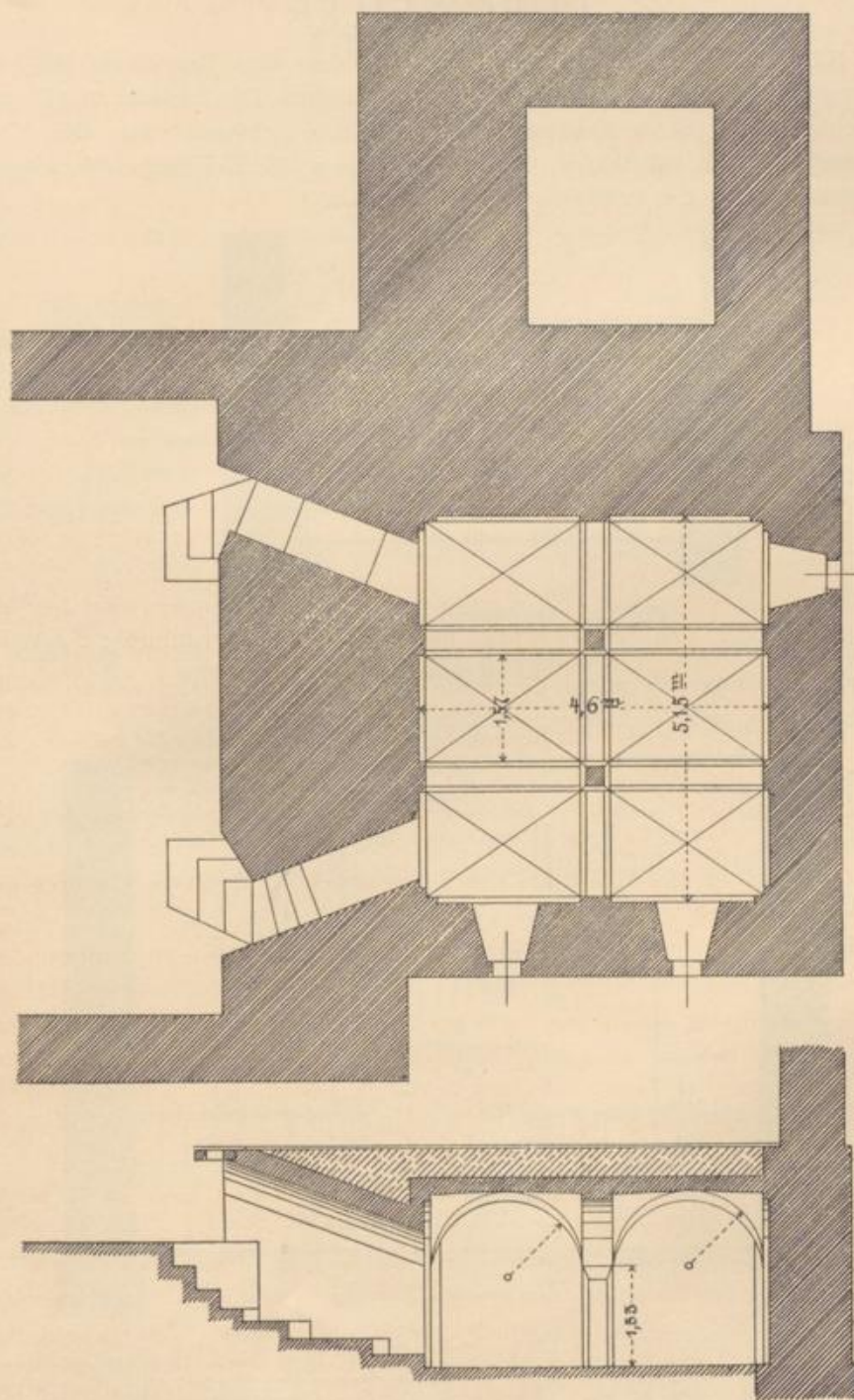
Fig. 109. Burgweiler, Krypta. Grundriss und Längenschnitt.
