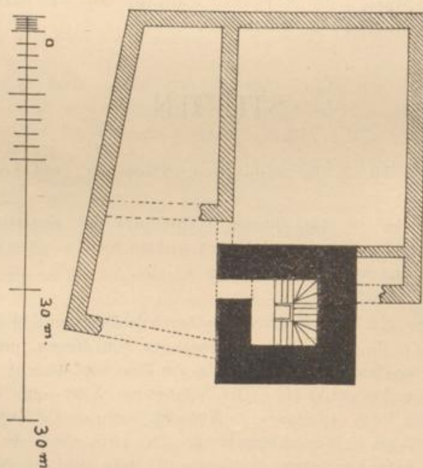
Fig. 22. Stetten. Grundriss des Neuhoewener Schlösschens.
