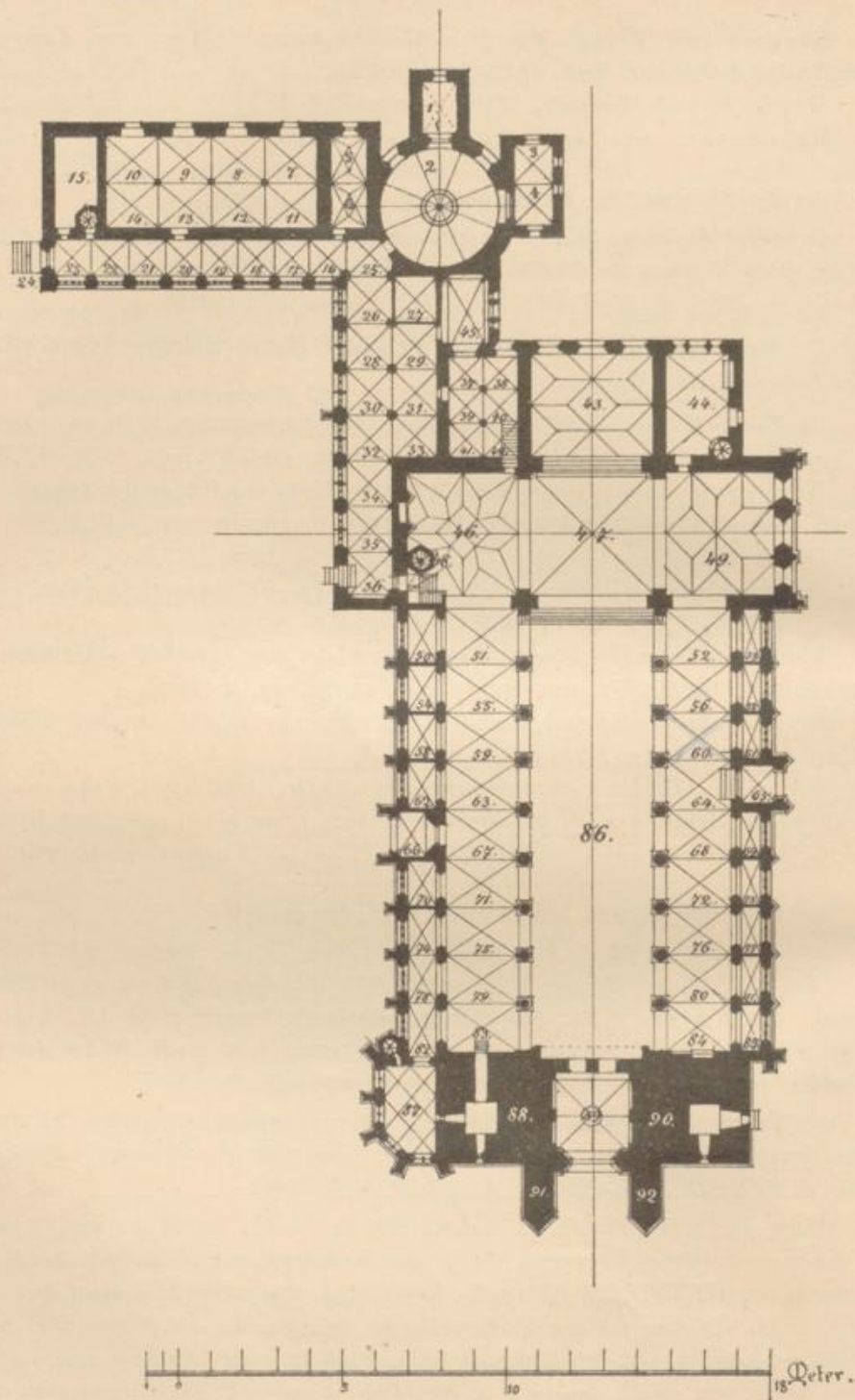
Fig. 33. Konstanz. Münster. Grundriss.
