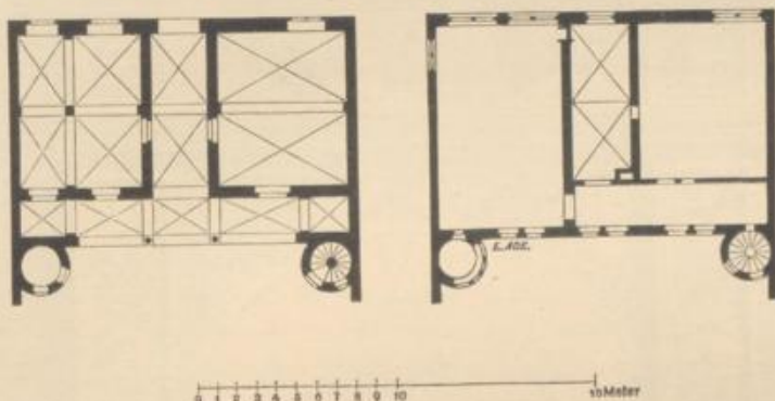
Fig. 72. Konstanz. Kanzleigebäude. Grundriss.
