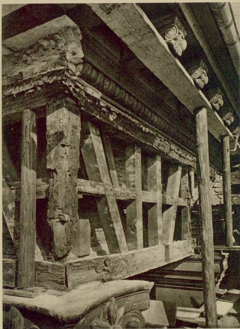
Abb. 13. Epistyl am Markgräfl. Palais in Karlsruhe. Aufgen. während der Ausbesserungsarbeiten i. J. 1925.
