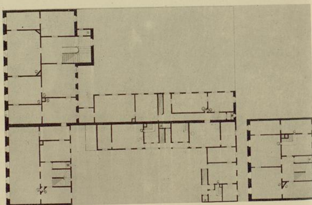
Abb. 54a: Grundriß des ersten Obergeschosses der Häuser Nr. 7 und 9 und Grundriß des zweiten Obergeschosses des Hauses Nr. 9 der Erbprinzenstraße
