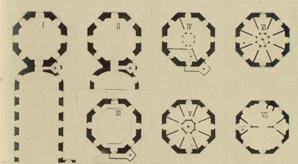
Abb. 33. Grundrisse des Karlsruher Schloßturmes.
