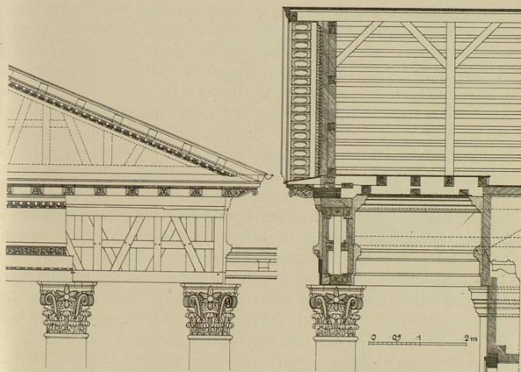
Abb. 10. Konstruktion des Epistyls am Markgräfl. Palais in Karlsruhe Aufgen. i. J. 1925.
