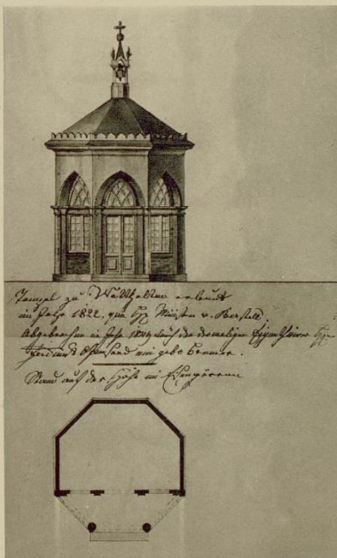
Abb. 62: Die Eremitage in Wattshalden von Joh. Ullrich 1822. Aus Ullrichs braunem Buch.
