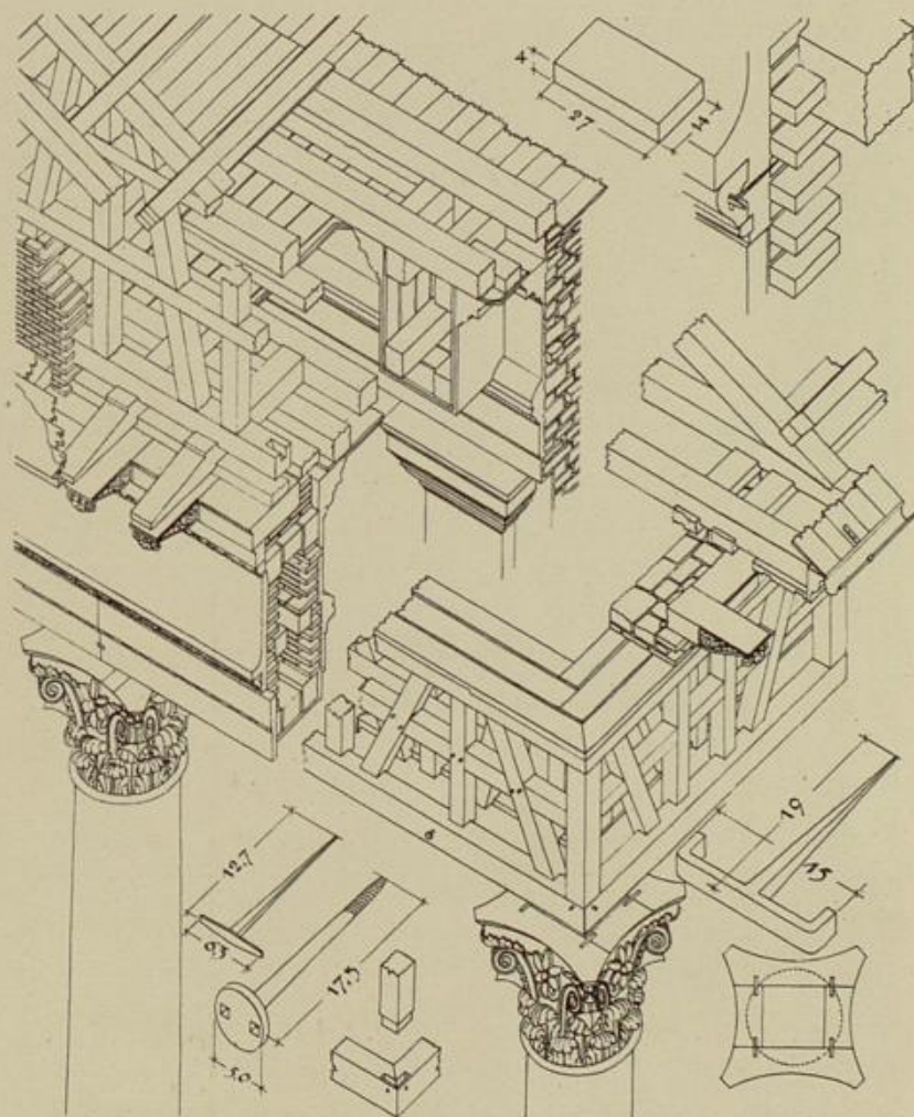
Abb. 11. Konstruktion des Epistyls am Markgräfl. Palais in Karlsruhe Aufgen. i. J. 1925.
