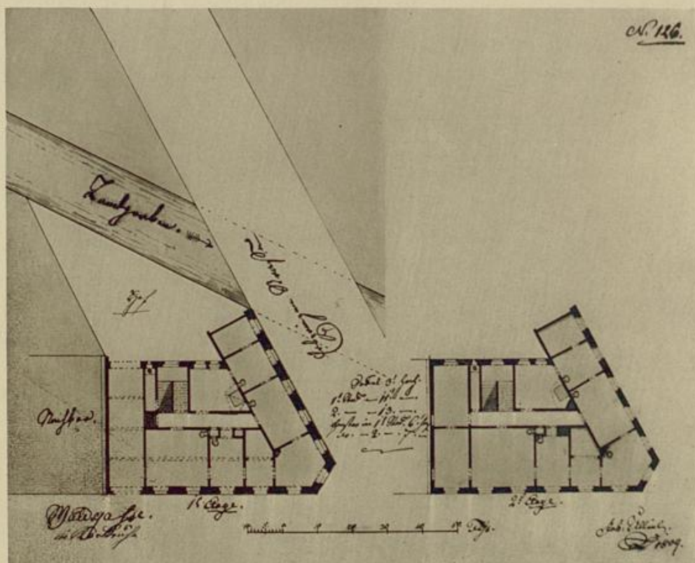
Abb. 83: Eckhaus des Anstreichers Kammerer, Waldstraße Nr. 53, erb. i. J. 1809. Plan aus dem sog. braunen Buch des Baumeisters Joh. Ullrich (cf. pag. 159/160).
