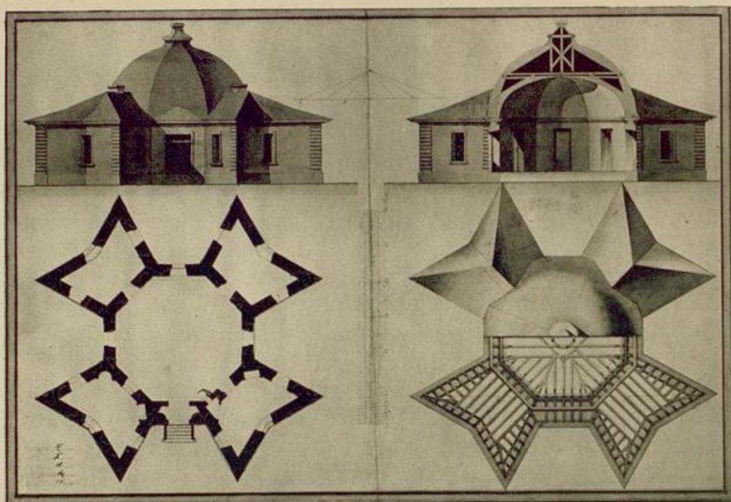
Abb. 31. Jagdhaus bei Dos. Originalplan ohne Beschriftung im Besitze des Bezirksbauamtes Baden-Baden.
