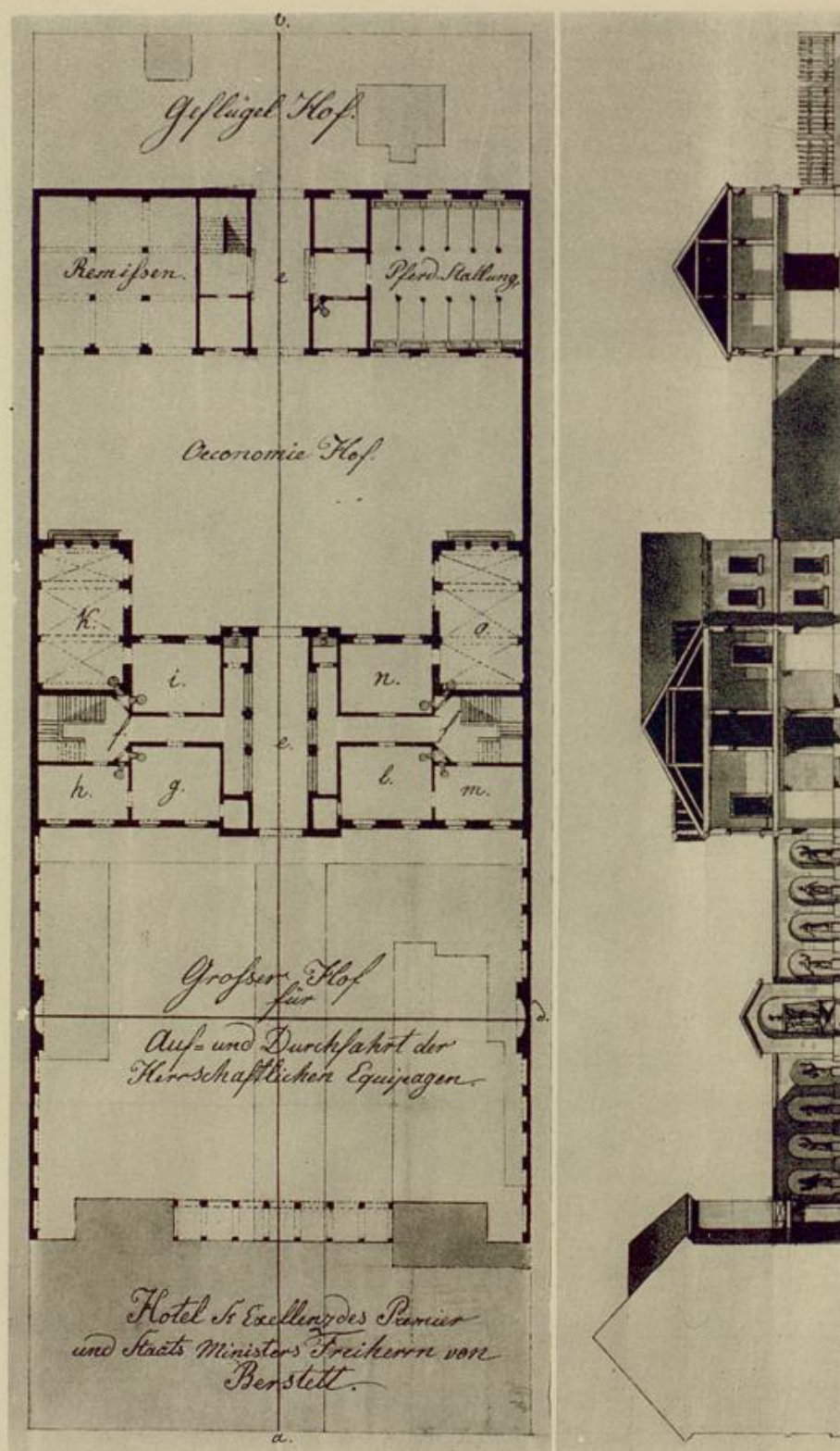
216b. 63: Vorschlag des Baumeisters Fischer für neue Hintergebäude auf den Grundstücken Nr. 7 und 9 der Erbprinzenstraße Aus den Akten Baudirektion Kof. 1. Fach 19. Fasc. 1.
