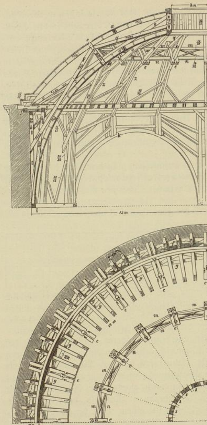
Abb. 135: Die Kuppelkonstruktion der Stephanskirche in Karlsruhe.
