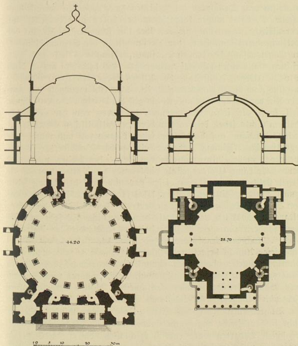
Abb. 133: Die Rotunde von St. Blasien. Abb. 134: Die Stephanskirche in Karlsruhe.
