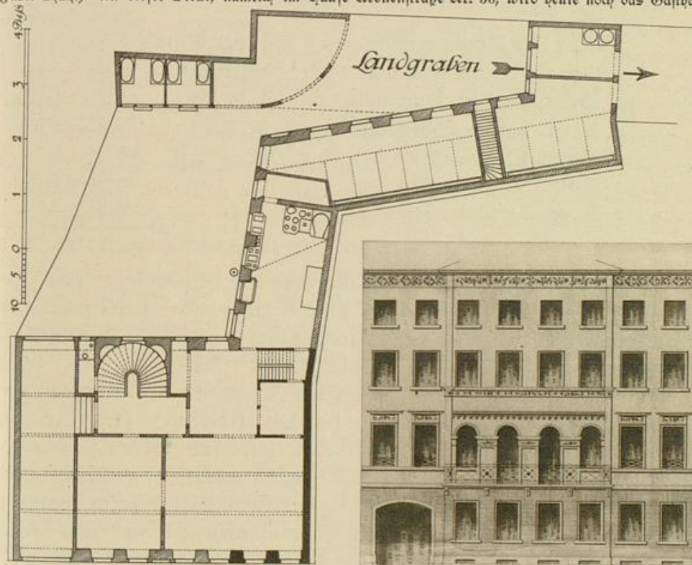
Abb. 157. Umbauprojekt des Hauses Kaiserstraße Nr. 187 vom Jahre 1856 nach einer Pause in den Akten „Polizei-Direktion Vauache“ fasc. 2656 G. L. A. Auf der Pause steht: „Entwurf und Arbeits-Plan zu einem Gast Hof für Herrn Hafner Salmen-Wirth — sect Friedrich Haug.“ Daneben Fassadenzeichnung aus denselben Akten ohne Beschriftung.
