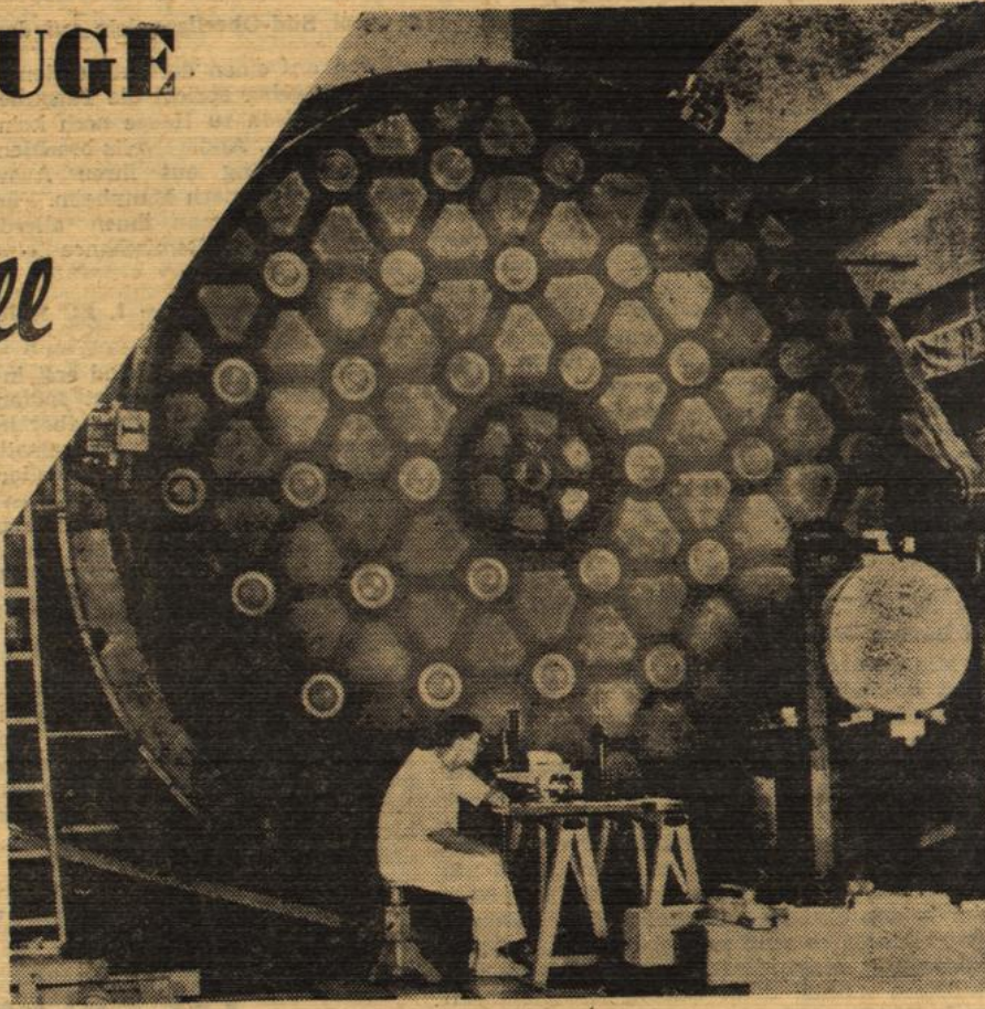
Ein Wissenschaftler überprüft den 5 Meter großen Spiegel.
