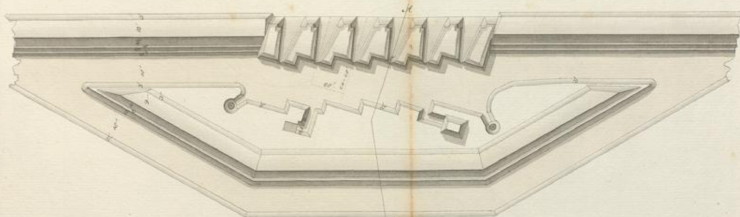
Plan der Batterie Grundriß von 6 parisiſchen Linien = 1 l
