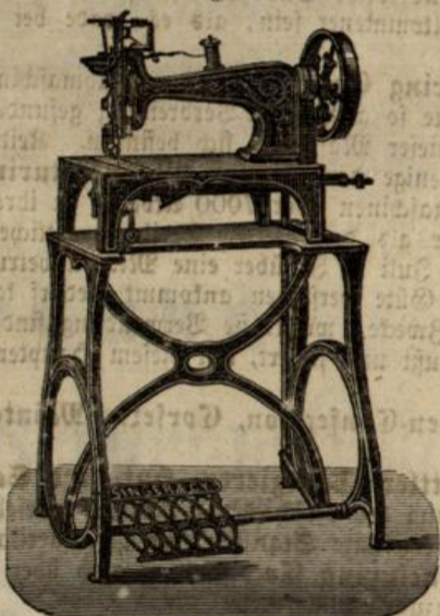
No. 2. Rollfuß-Maschine für Perlstich und alle Arten Schuhmacher-Arbeiten.
