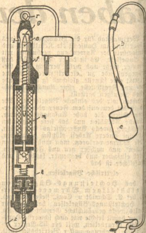
Gaszündvorrichtung Tauchflöter
