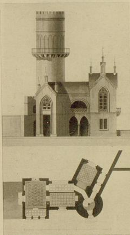
Abb. 54. Grundriß und Aufriß des sog. gotischen Thurmes im Erbprinzen-garten Unbeschrifteter Plan im G.E.N.
