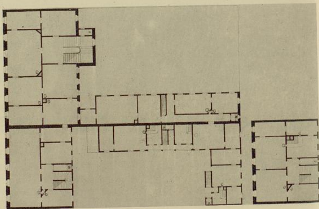
Abb. 54a: Grundriß des ersten Obergeschosses der Häuser Nr. 7 und 9 und Grundriß des zweiten Obergeschosses des Hauses Nr. 9 der Erbprinzenstraße Aus den Akten Baudirektion Kast. 1, Fach 19, Fasc. 1.
