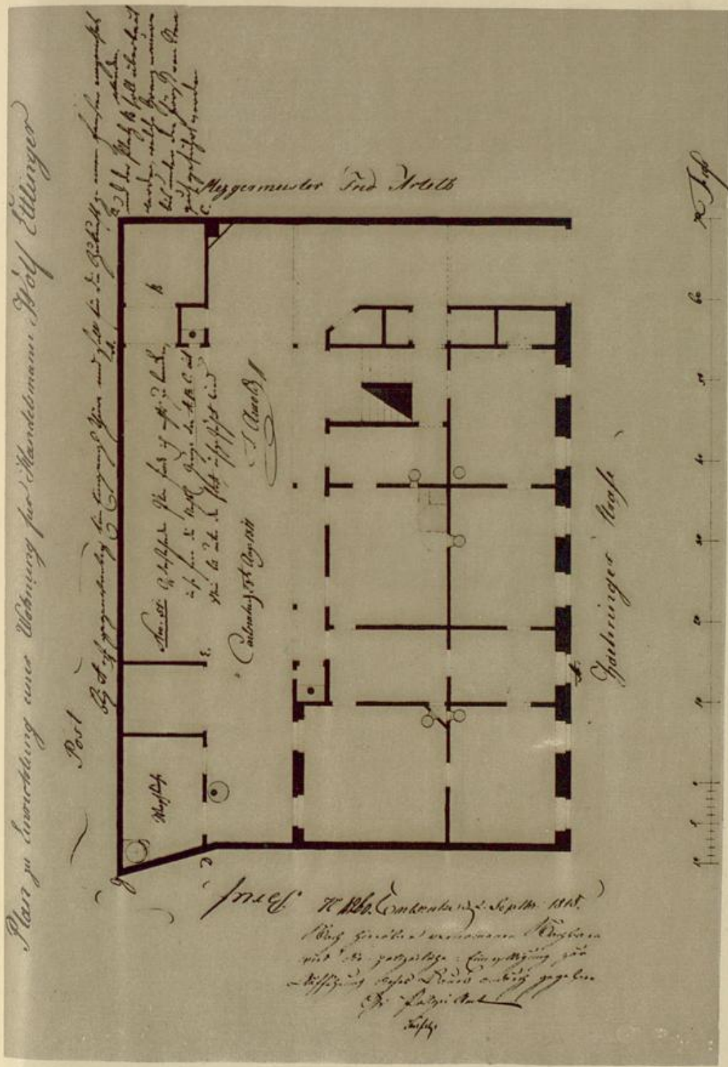
Abb. 99: Fähringerstraße Nr. 55, Grundriß
