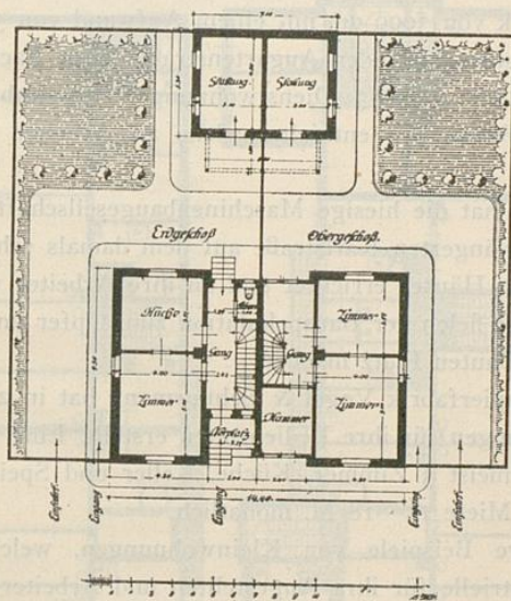
Abb. 6 Städt. Arbeiterwohnhaus Karlsruhe. 1911.
