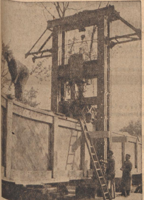
Die größte Holzbrücke der Welt wurde zwischen Kehl und Straßburg durch Gauleiter Robert Wagner dem Betrieb übergeben. Die Brücke ist eine neuartige Konstruktion, deren wissenschaftliche Erforschung in dem Lehrstuhl für Brücken der Techn. Hochschule in Karlsruhe in Verbindung mit der Versuchsanstalt Holz, Stein, Eisen unter Leitung von Prof. Dr.-Ing. Gaber erfolgte.
