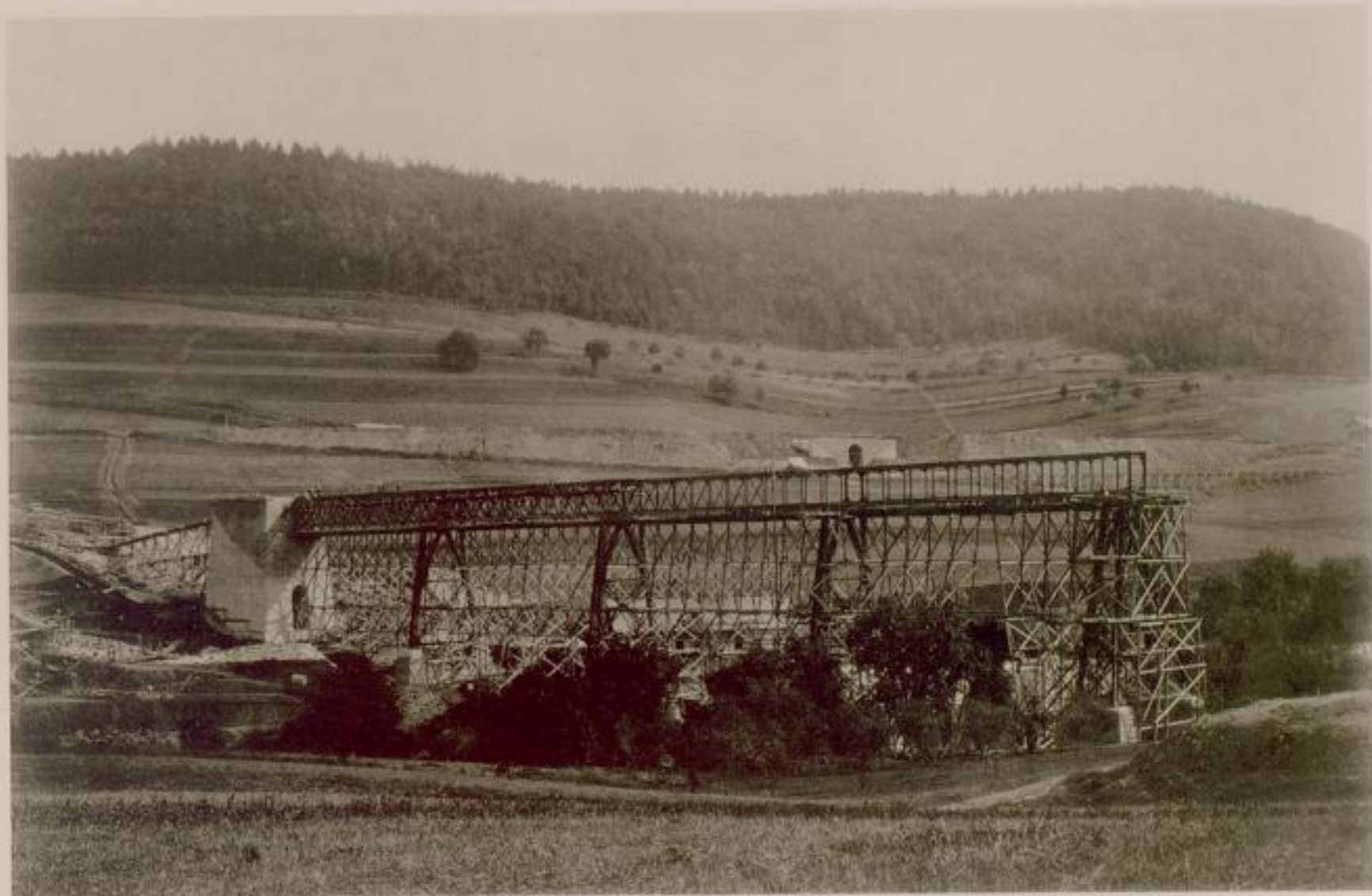
GERÜST FÜR DEN EFFENHOFENER THALÜBERGANG.
