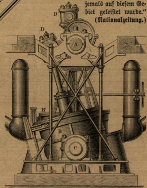
Destillierende Swillingsschiffsmaschine.
