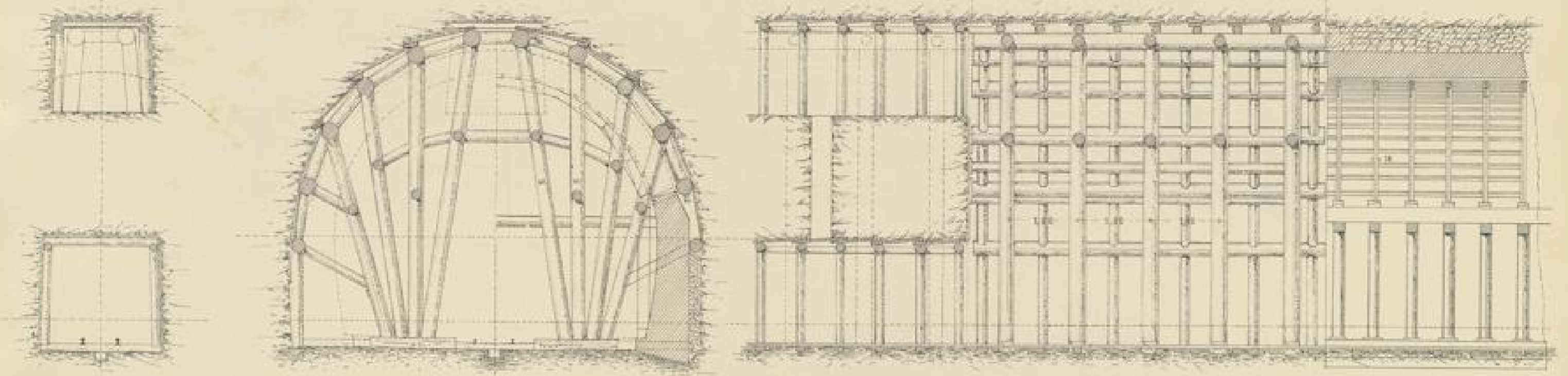
Fig. 1 für Mauerungsprofil 5.
