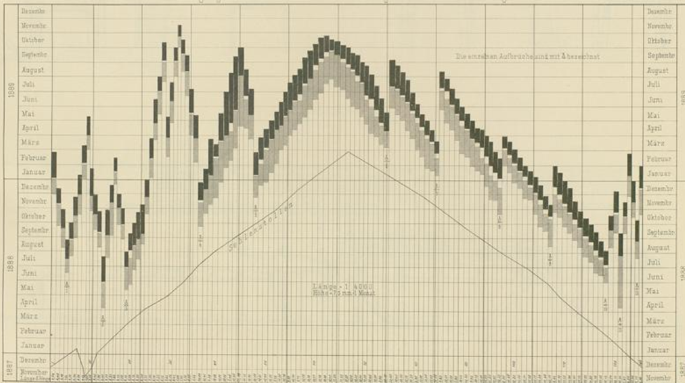
Fortgang des Ausbruches u der Mauerung der einzelnen Gewölbringe
