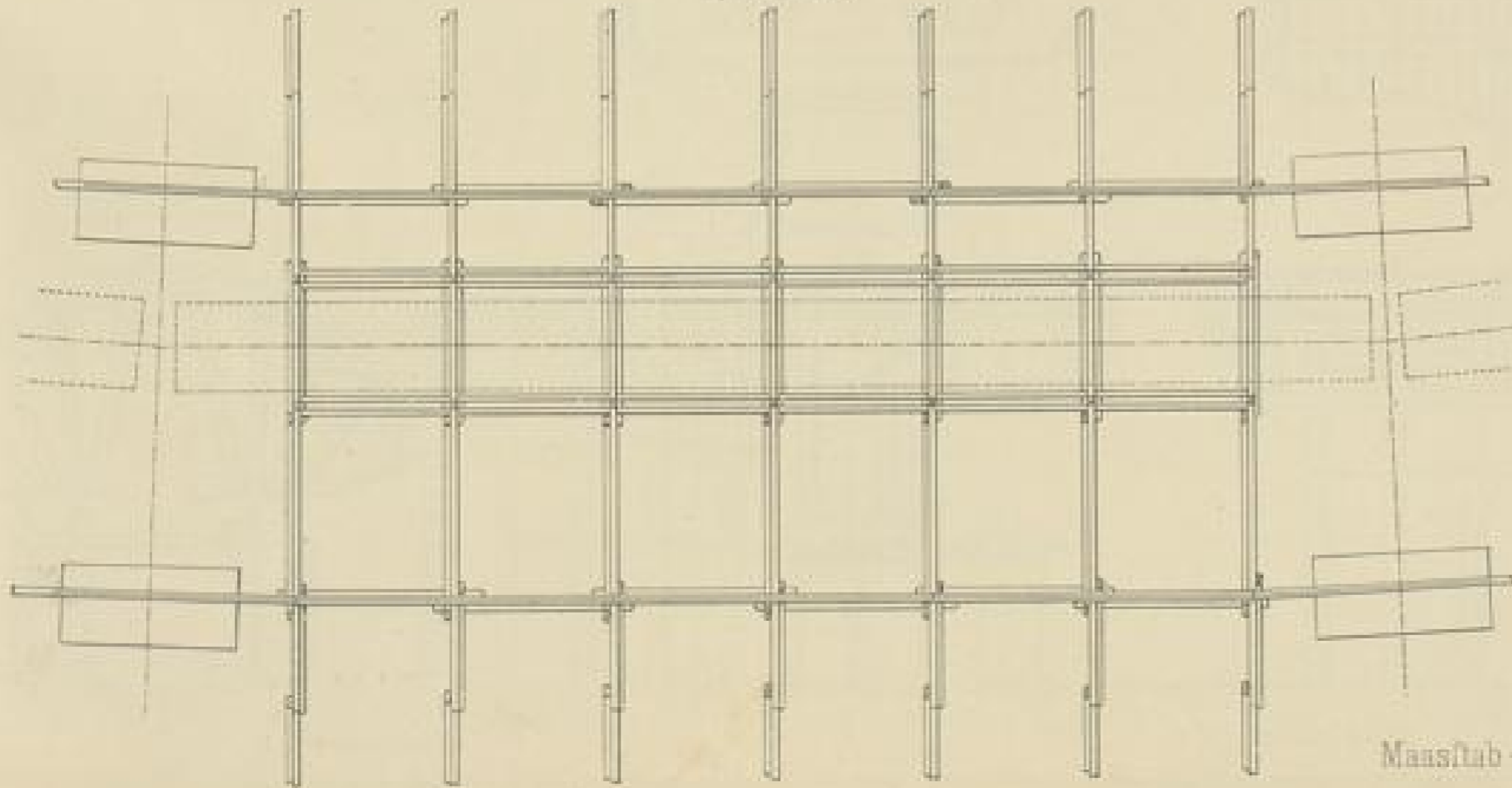
Grundriß
