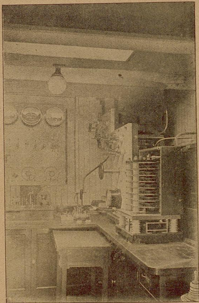
Funkenstation der „Hitachi Maru“.
