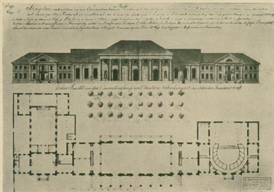
Weinbrenners Originalentwürfe für das Conversationshaus; unterer Entwurf unausgeführt.
