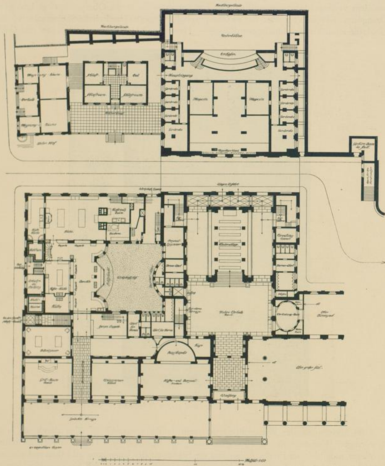
Der Neubau: Erdgeschoßgrundriß.
