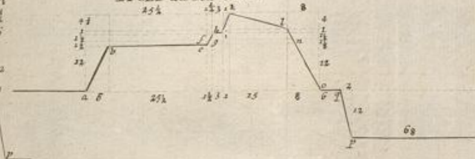
Fig. XI. Profil du Ravelin
