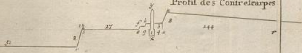
Fig. XIII. Profil des Contrescarpes
