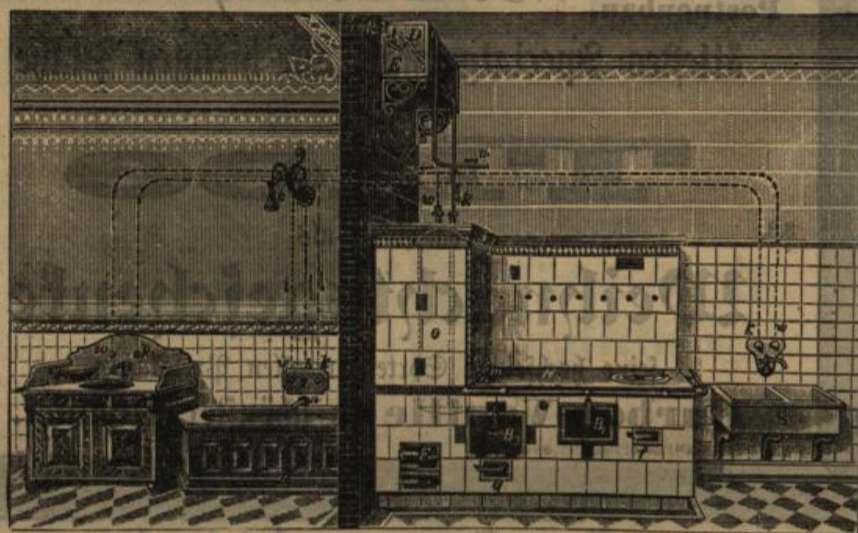
Warmwasser-Bereitung vom Küchenherd aus für Bade-, Toilette- und Spülzwecke.
