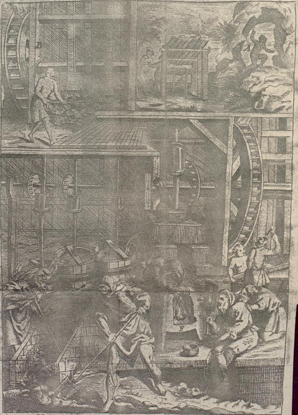
A: Das Berg- und Ziehwerk B: Die Pochmühle C: Die Waschmühle D: Die Sicher oder Waschtrüge E: Der Röstofen F: Der Schmelzofen.
