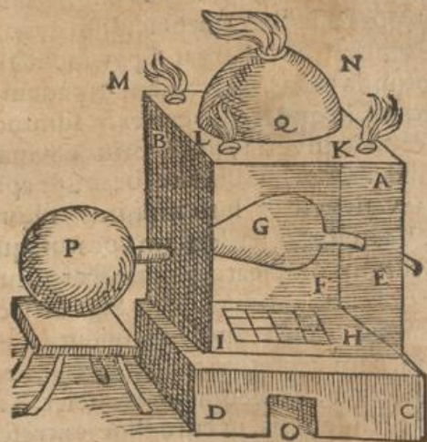
Fornax, A. B. C. D. Ferrum fulciens vas cavum, E. F. Ampulla, G. Testudo, Q. Crates ferrea, H. I. Quatuor infumibula, K. L. M. N.
