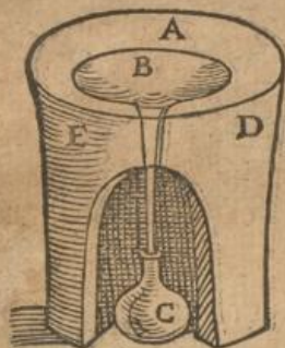
A. Vacuum cinere replendum, B. Vas distillatorium. D. E. Fornax. C. Receptaculum.
