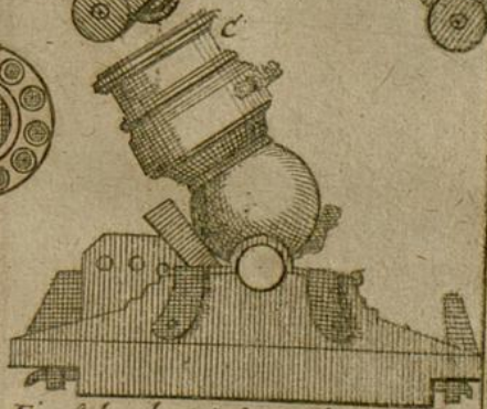
Ein stehender Mörser nach der Französischen facon.
