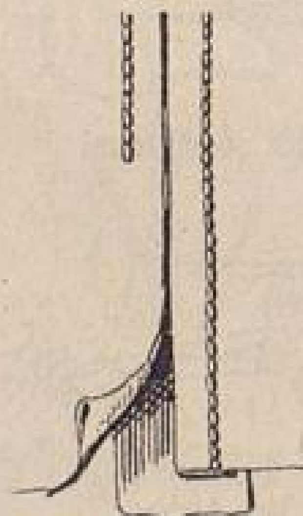
Abb. 8. Kellernaht.
