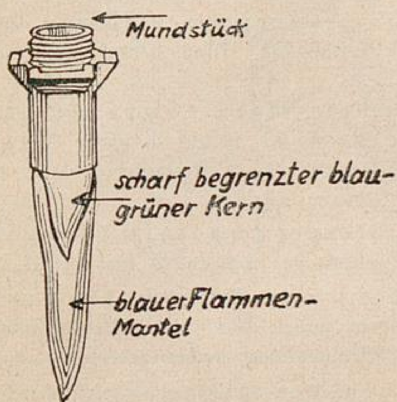
Richtig einregulierte Gasflamme
