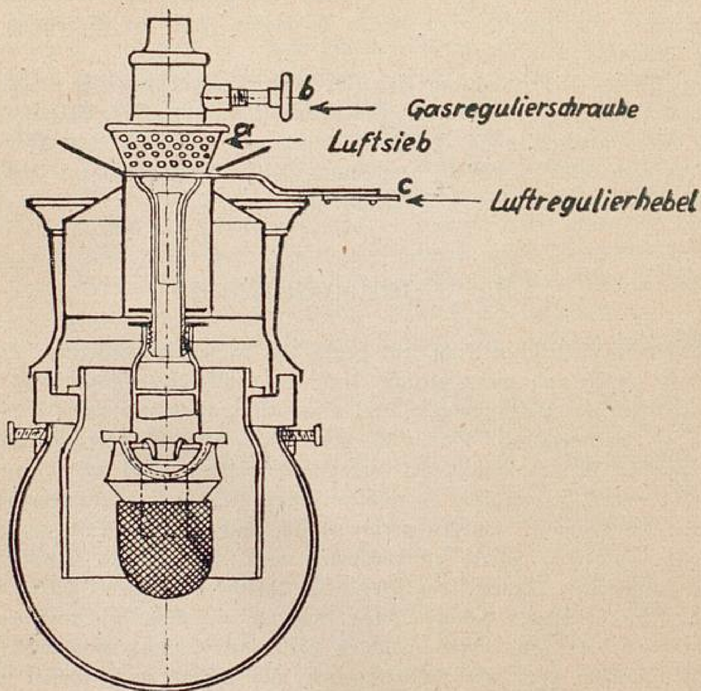
Gaslampe mit Hängeglühlicht
