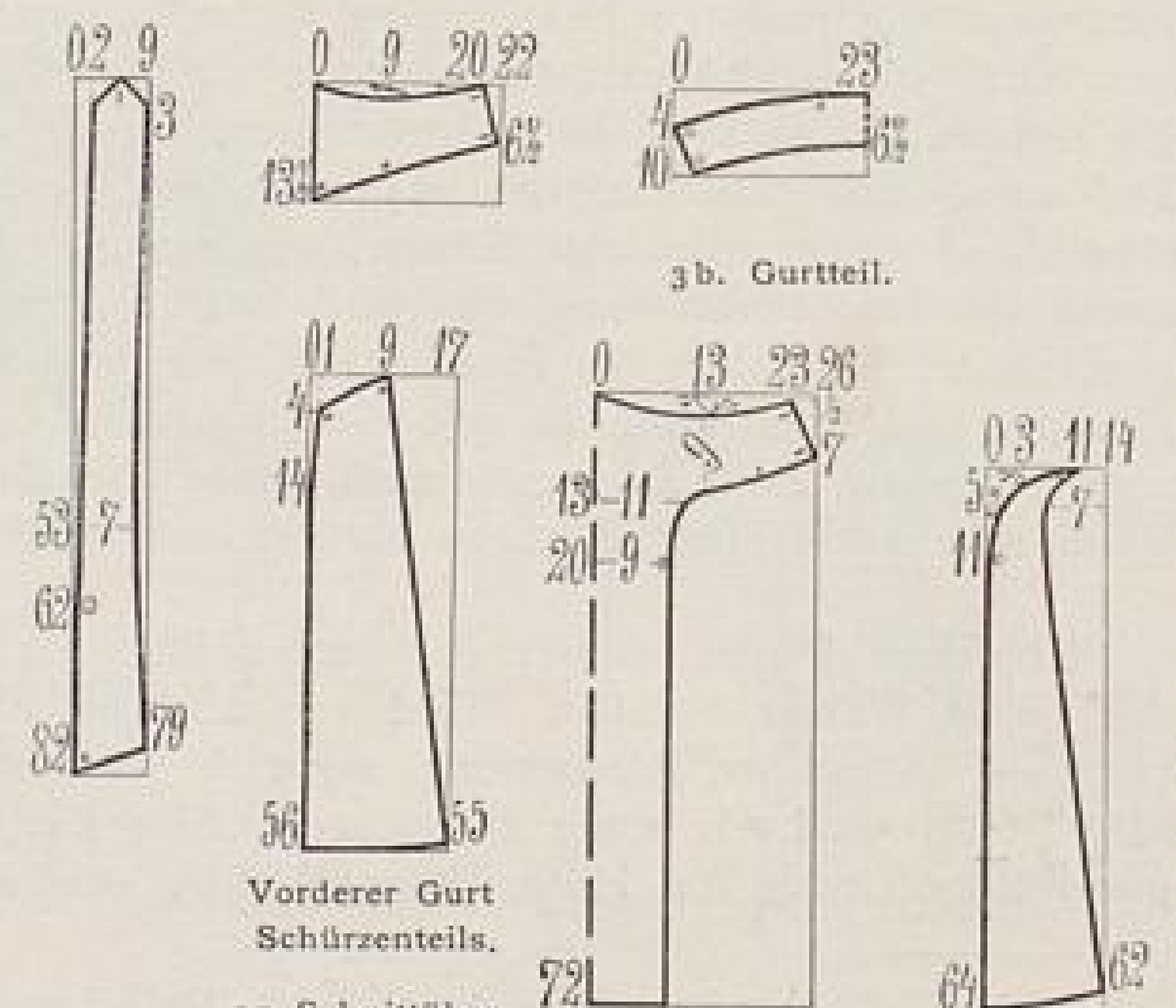
3a. Schnittübersicht zur Schürze Abb. 3. 4a. Schnittübersicht zur Schürze (Abb. 4). Vorderer Gurt Schürzenteils. Vorderbahn. Seitenbahn.
