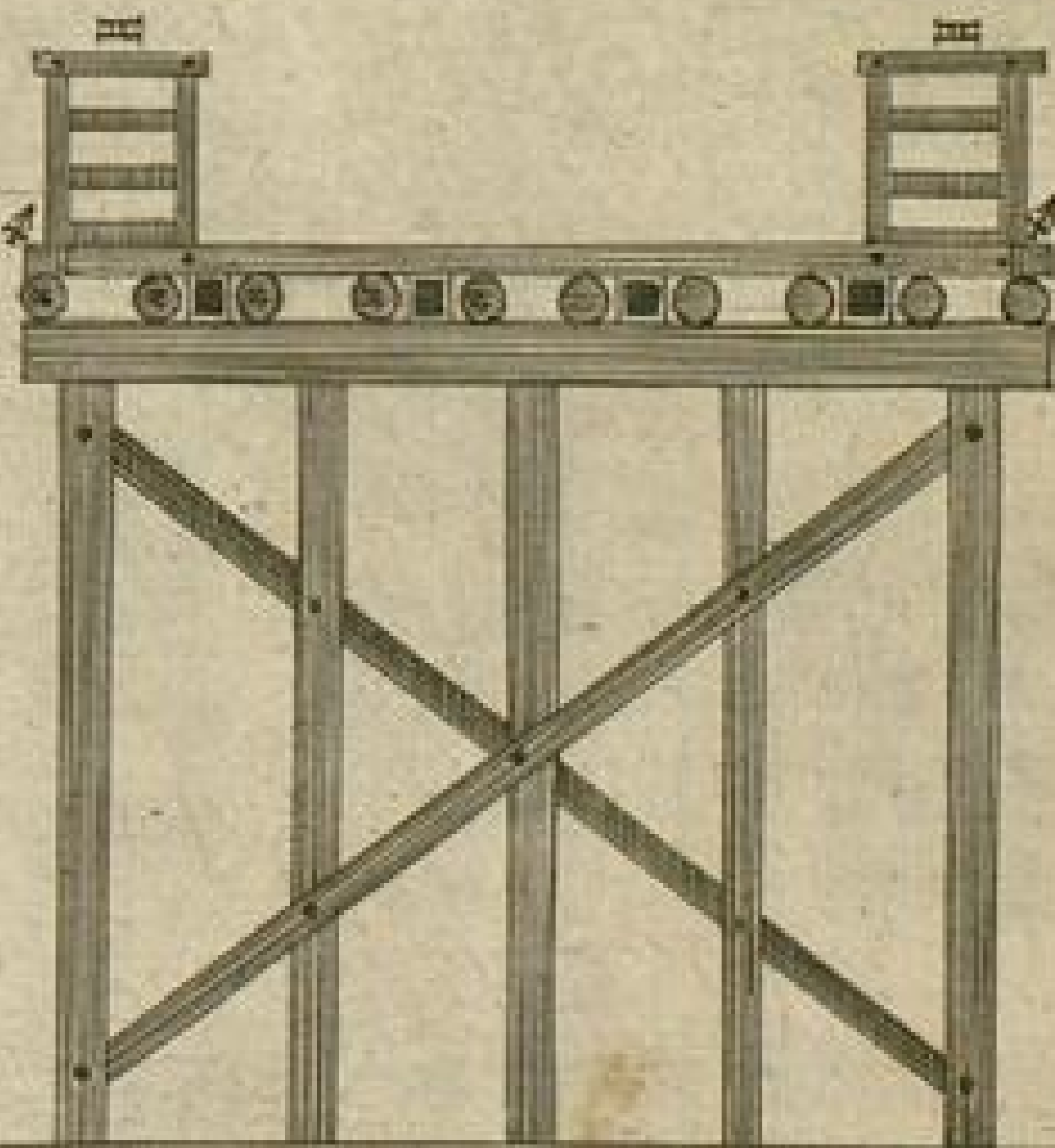
Profil eines Jochs
