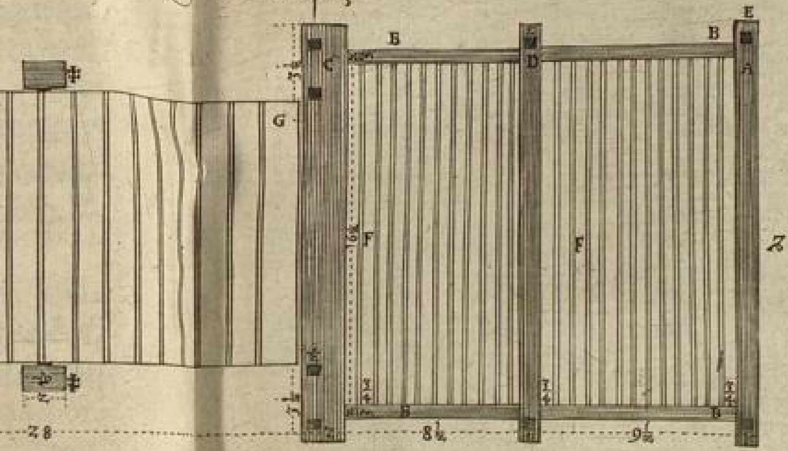
Plagbrücken Grundriß
