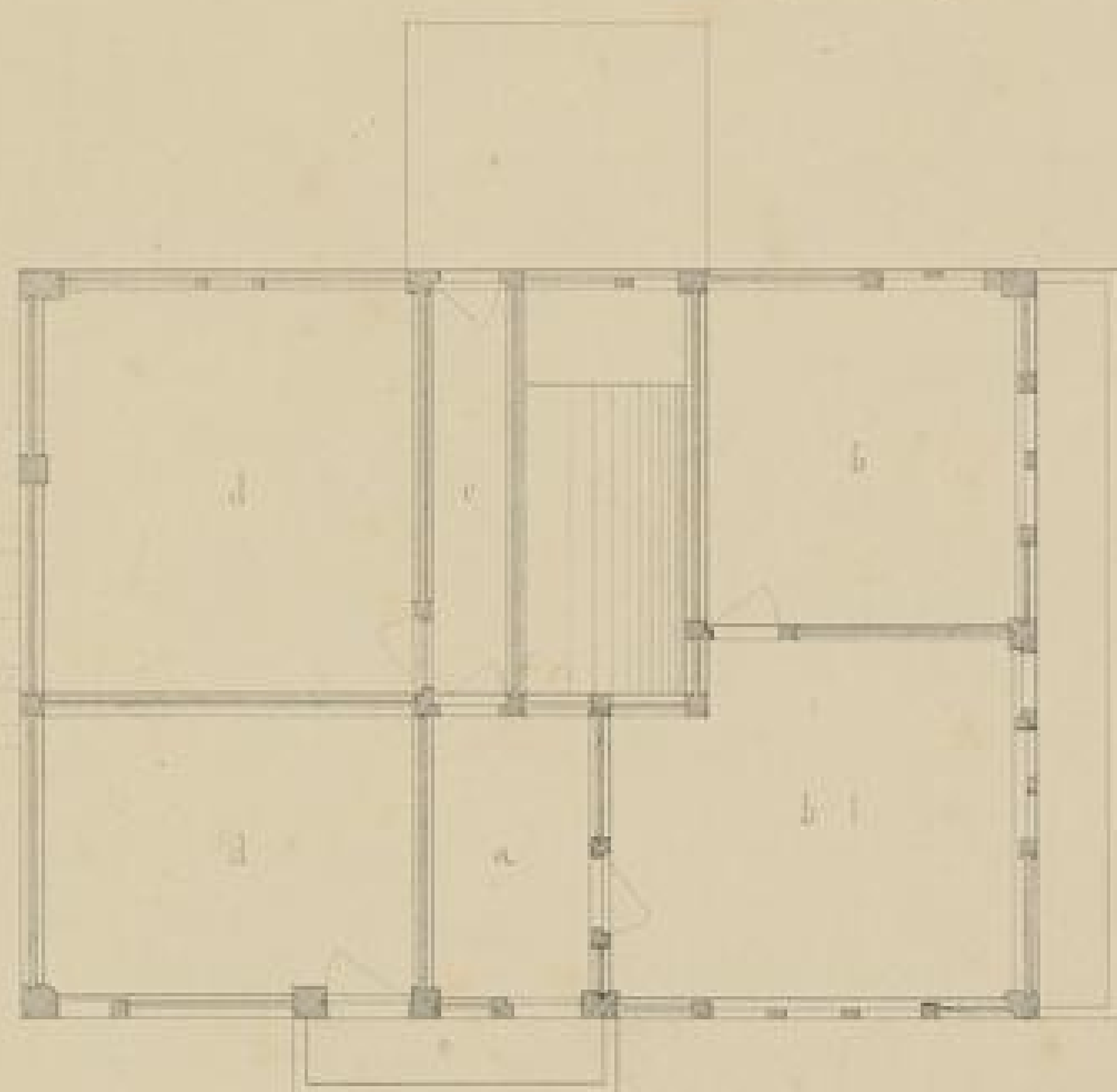
Grundriss des II. Stockes.
