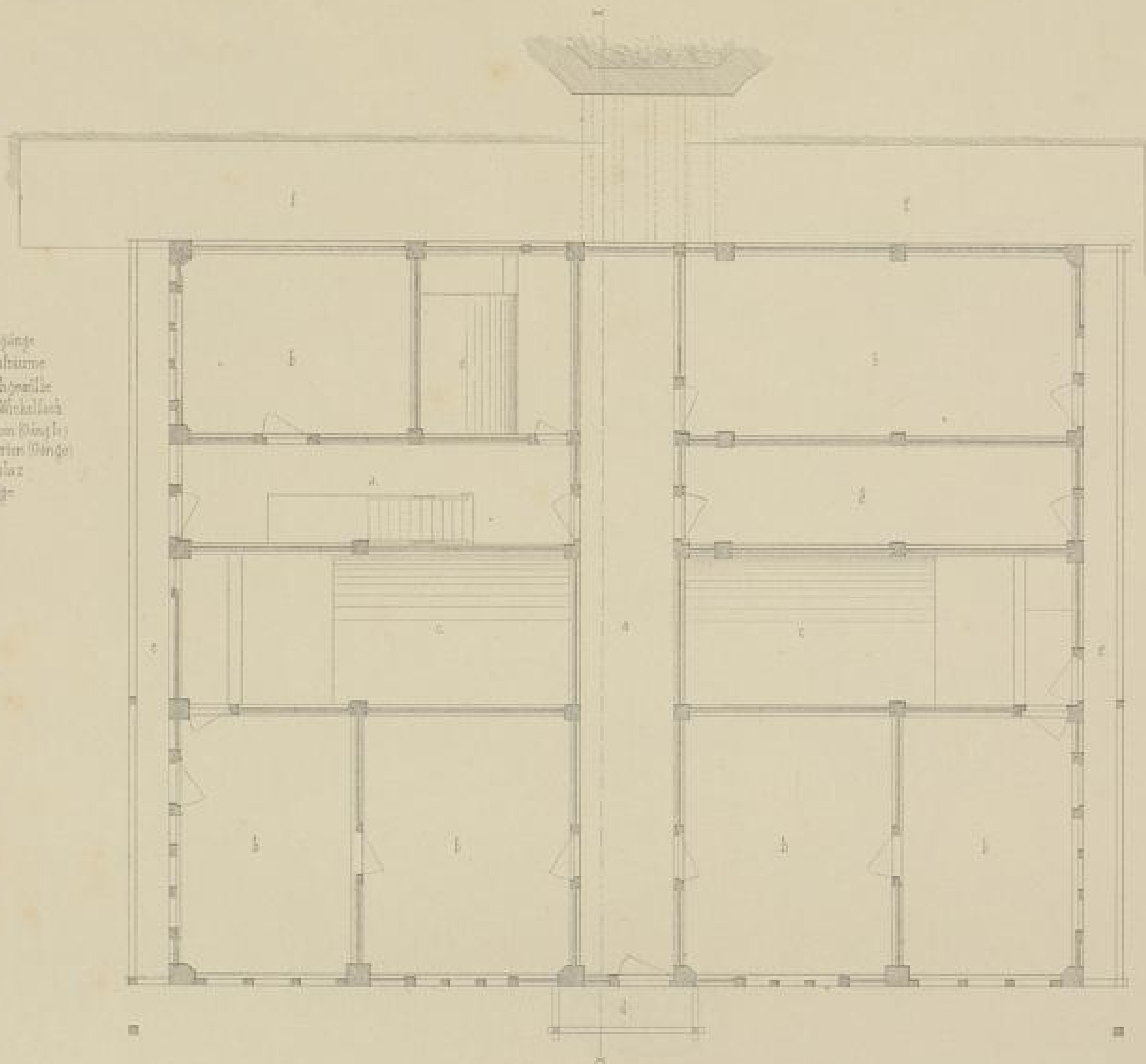
Grundriss des I Stockes
