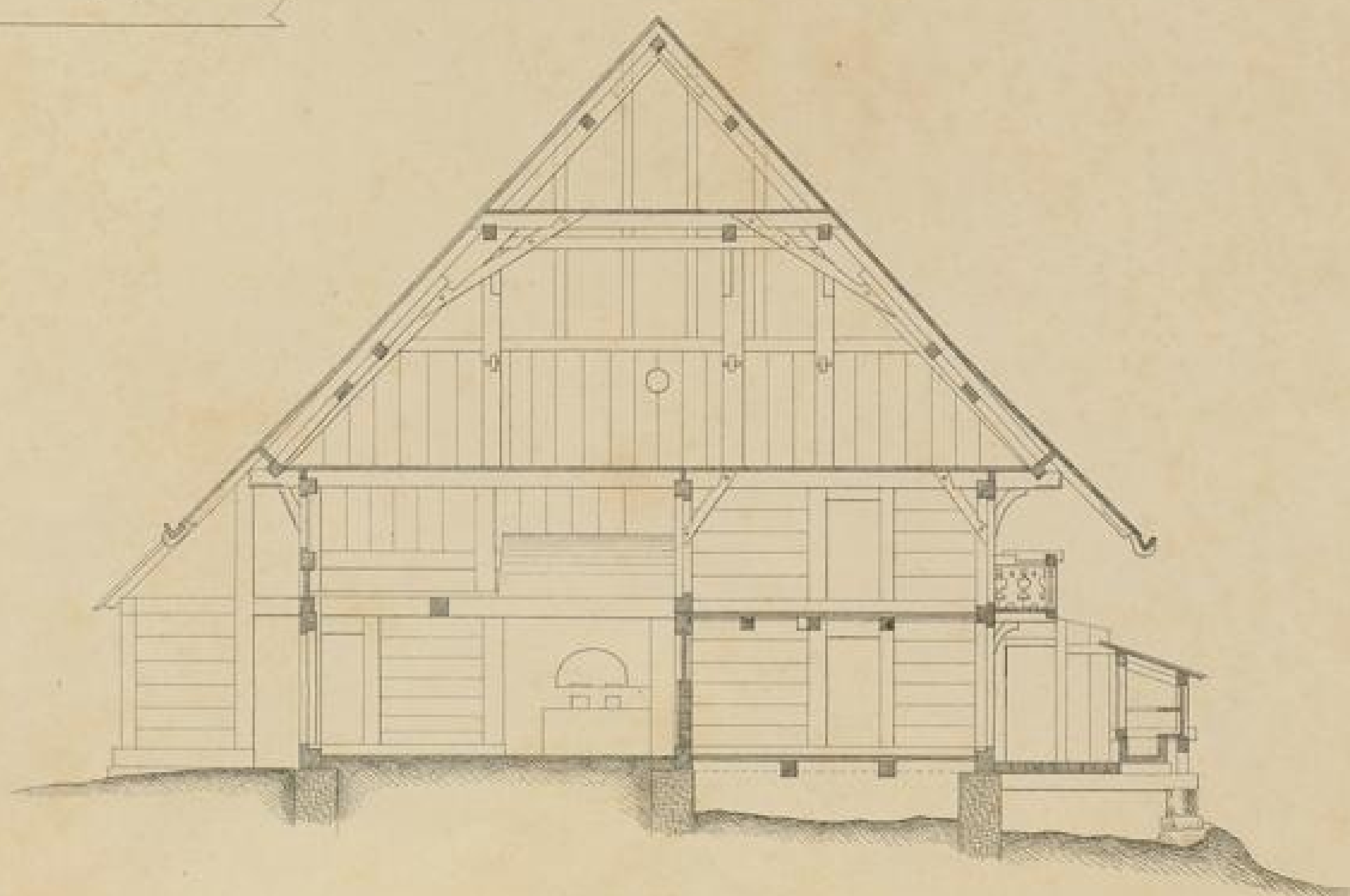
Querschnitt II nach v/x
