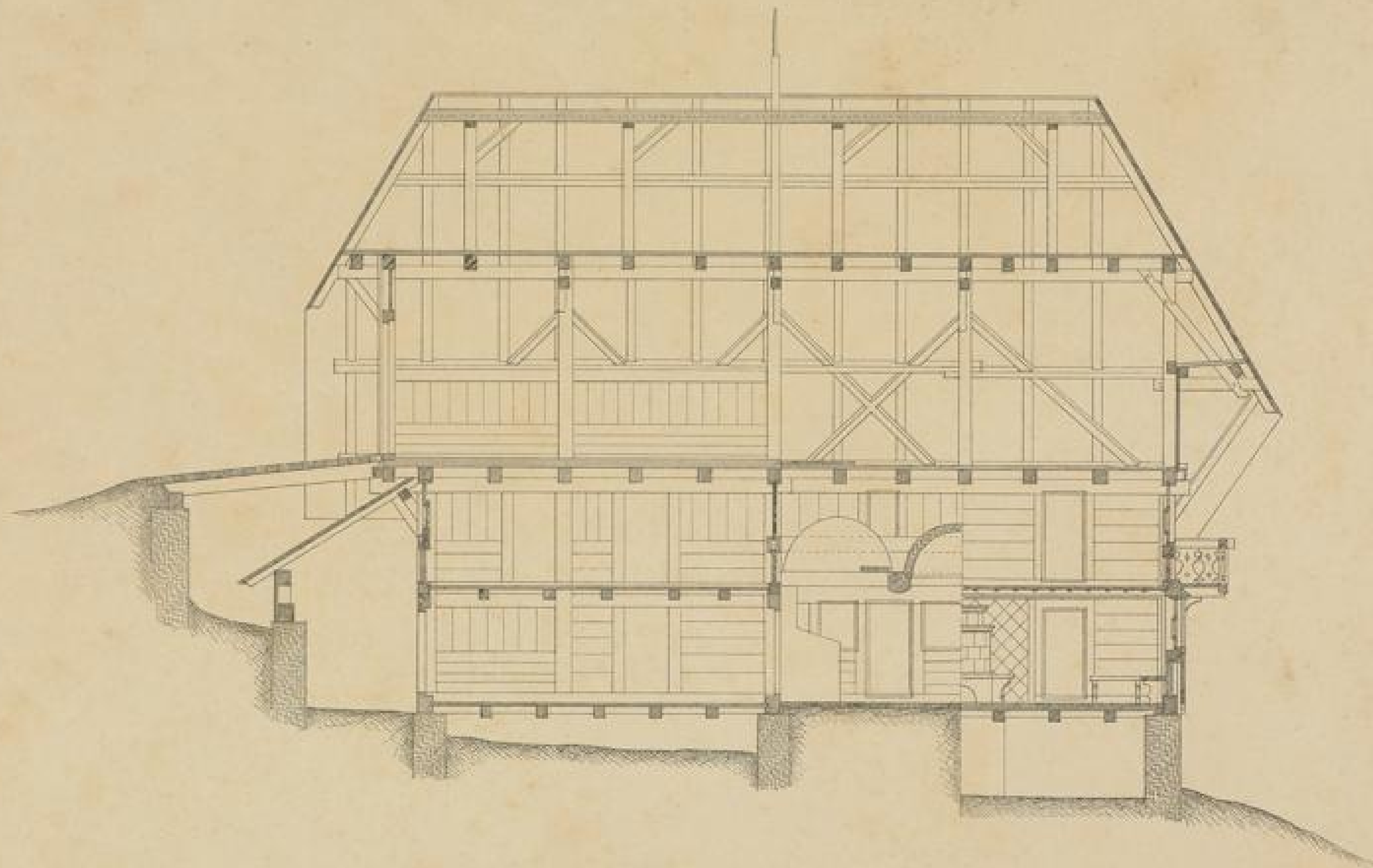
Längsdurchschnitt nach pp
