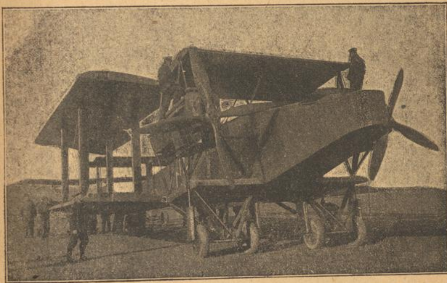
Englisches Großflugzeug, das unversehrt in deutsche Hände fiel. Das Flugzeug ist 30 m breit, 20 m lang und 6 1/2 m hoch, hat 2 Motoren und 3 Maschinengewehre; Besatzung 5 Mann.
