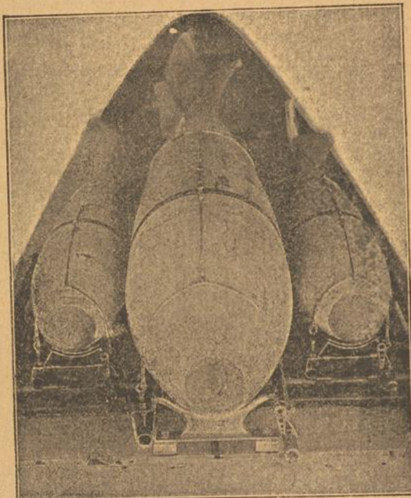
Deutsche Fliegerbomben im Gewicht von 1 und 6 Ztr. in der Aufhängevorrichtung unter dem Flugzeuge.
