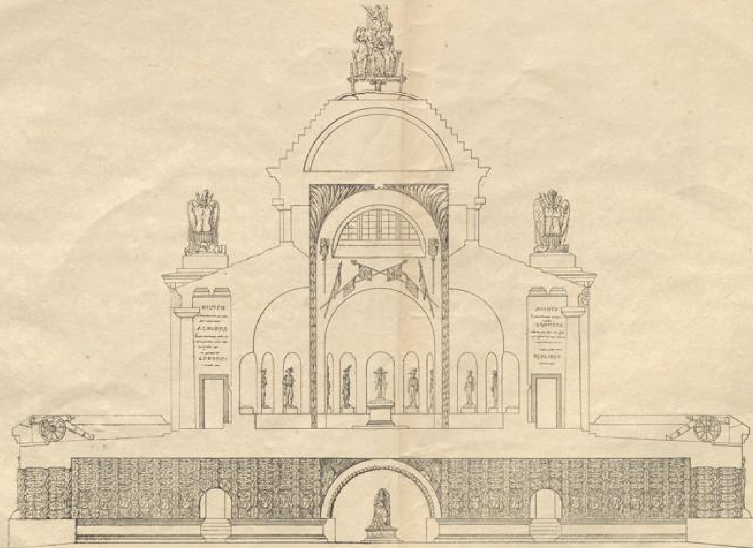
Durchschnitt durch die Mitte des ganzen Monuments auf das Leipziger Schlachtfeld.
