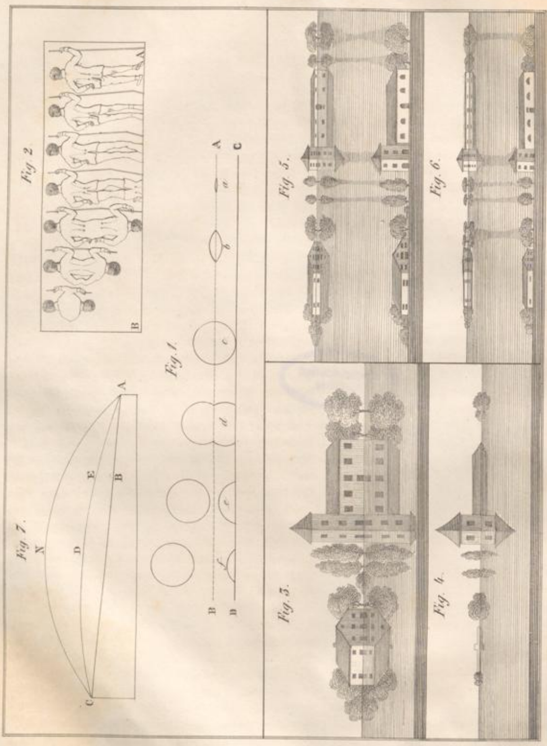
Luftspiegelungen.
