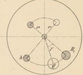
Vorderrad Fig. 4.
