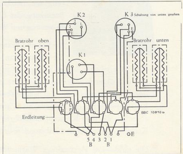
Dreiplattenherd Abb. 1
