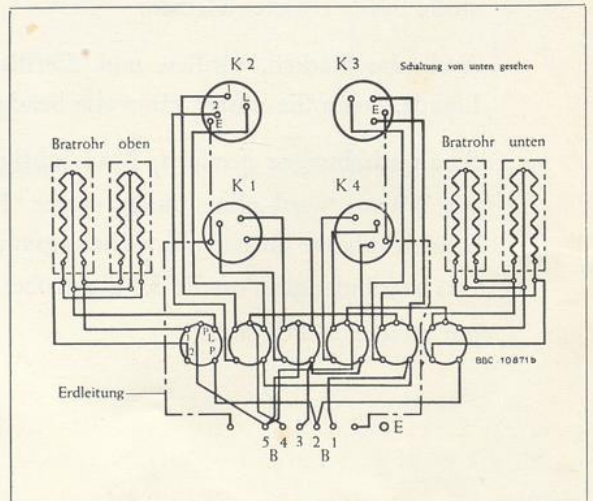
Vierplattenherd Abb. 2
