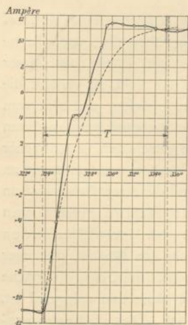
Fig. 22. Aufgenommene und konstruierte Kurzschlussstromkurve.
