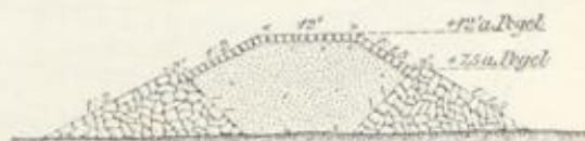
Abb. 24. Querschnitt des im Jahre 1868 begonnenen Parallelwerks an der Schottel.
