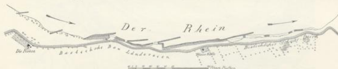
Abb. 59. Uferdeckung vor dem Bislicher Schaardeich, Zustand im Jahre 1779 (nach Eversmann).
