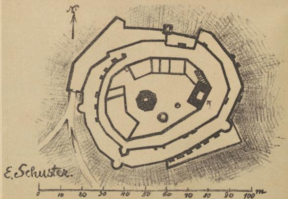
Grundriß der Ruine Steinsberg.
