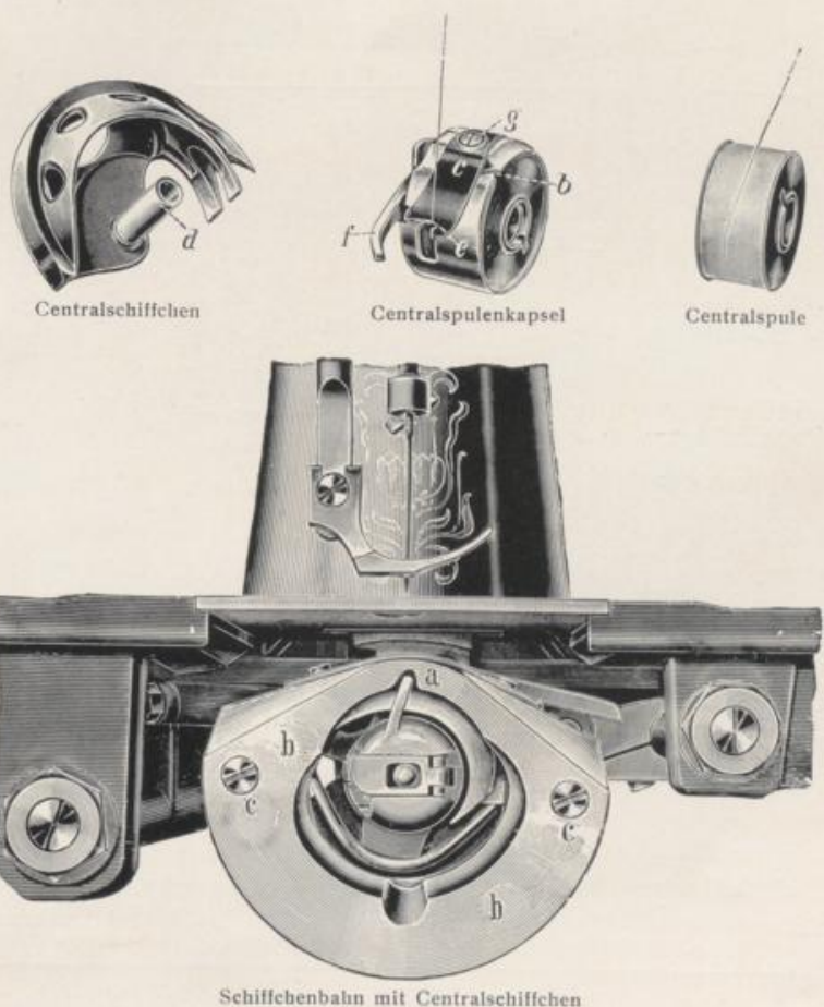
Schiffchenbahn mit Centralschiffchen
