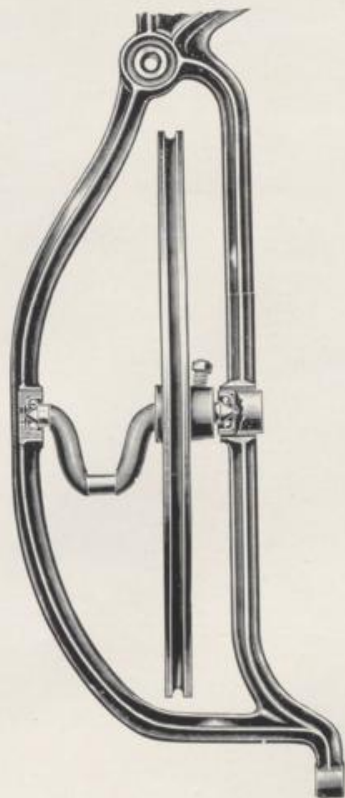
Querschnitt der Kugellager-Anordnung des modernen Gestelles M, auf welchem die Erda- u. Frigga-Maschinen geliefert werden
