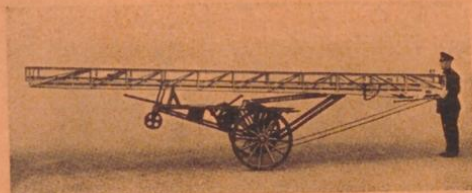
Metz - Patent - Zweiradleitern von 8—24 Meter Steighöhe, in Ganzstahlausführung oder Holz-stahlarmiert
