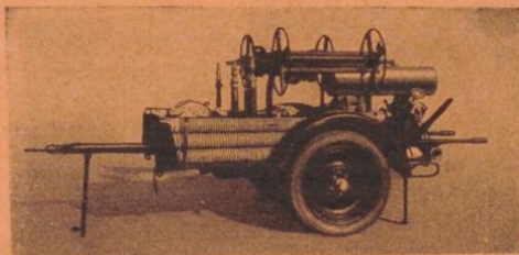
Metz-Motorfeuerspritzen, trag- und fahrbar, Motor wasser- oder luftgekühlt, auf Wunsch mit Schaum- löscheinrichtung, Transportwagen offen oder geschlossen
