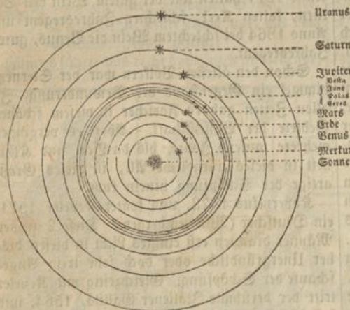
Einfachste Darstellung des Umlaufs der 11 bekanntesten Planeten um die Sonne.
