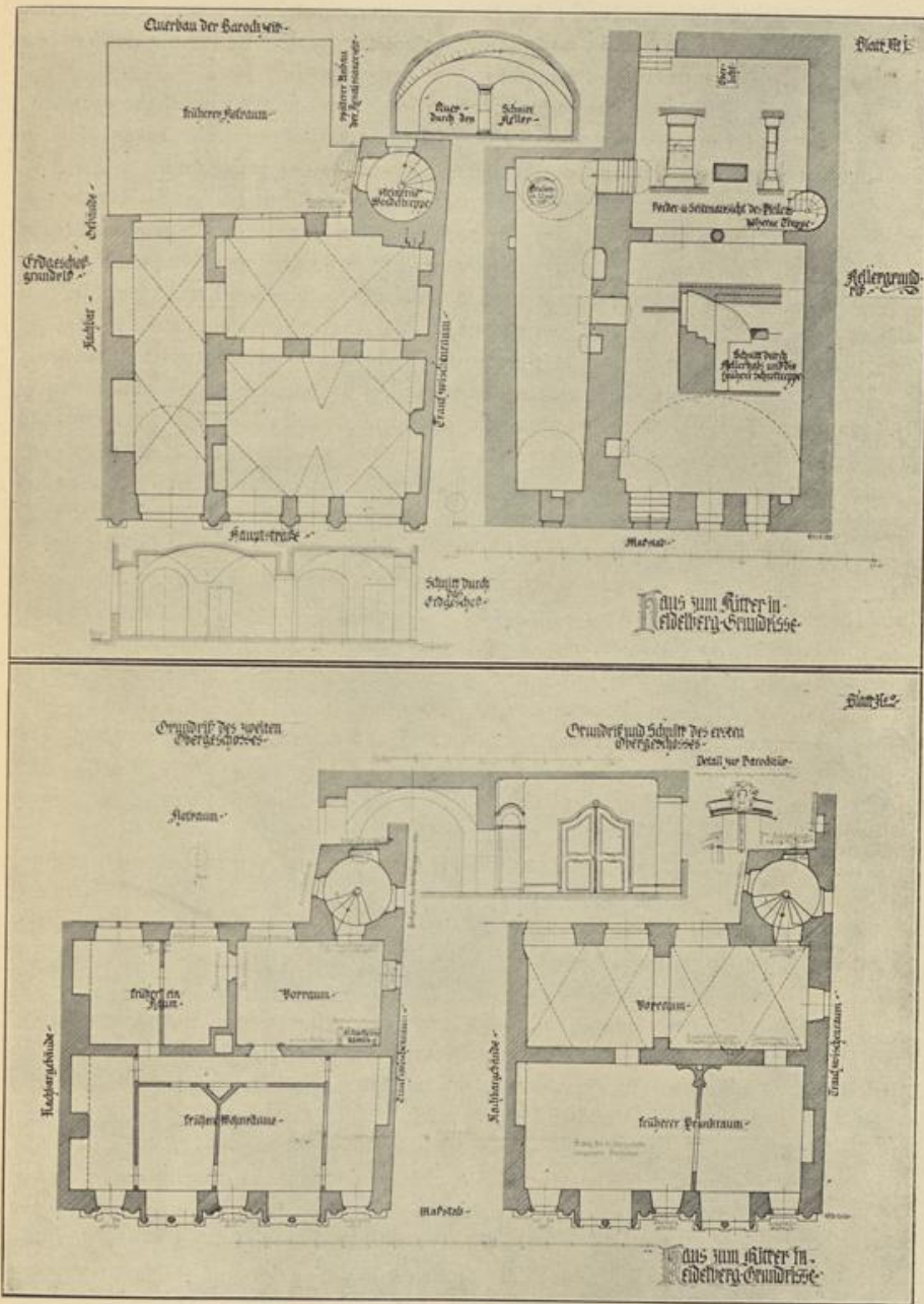
Fig. 207. Grundrisse der Häuser „Zum Ritter“.
