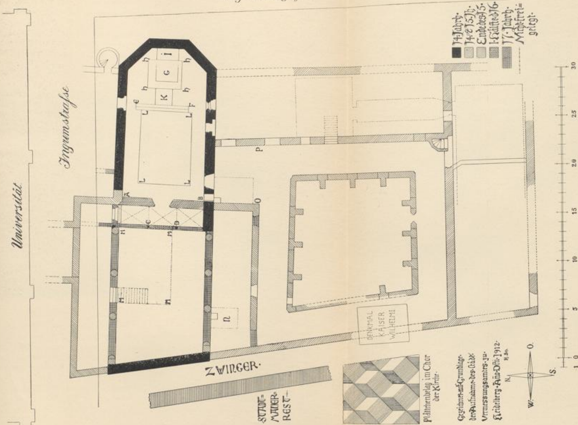
Fig. 237. Grundriß des Augustinerklosters zu Heidelberg. (Nach den Ausgrabungen i. J. 1912.)
