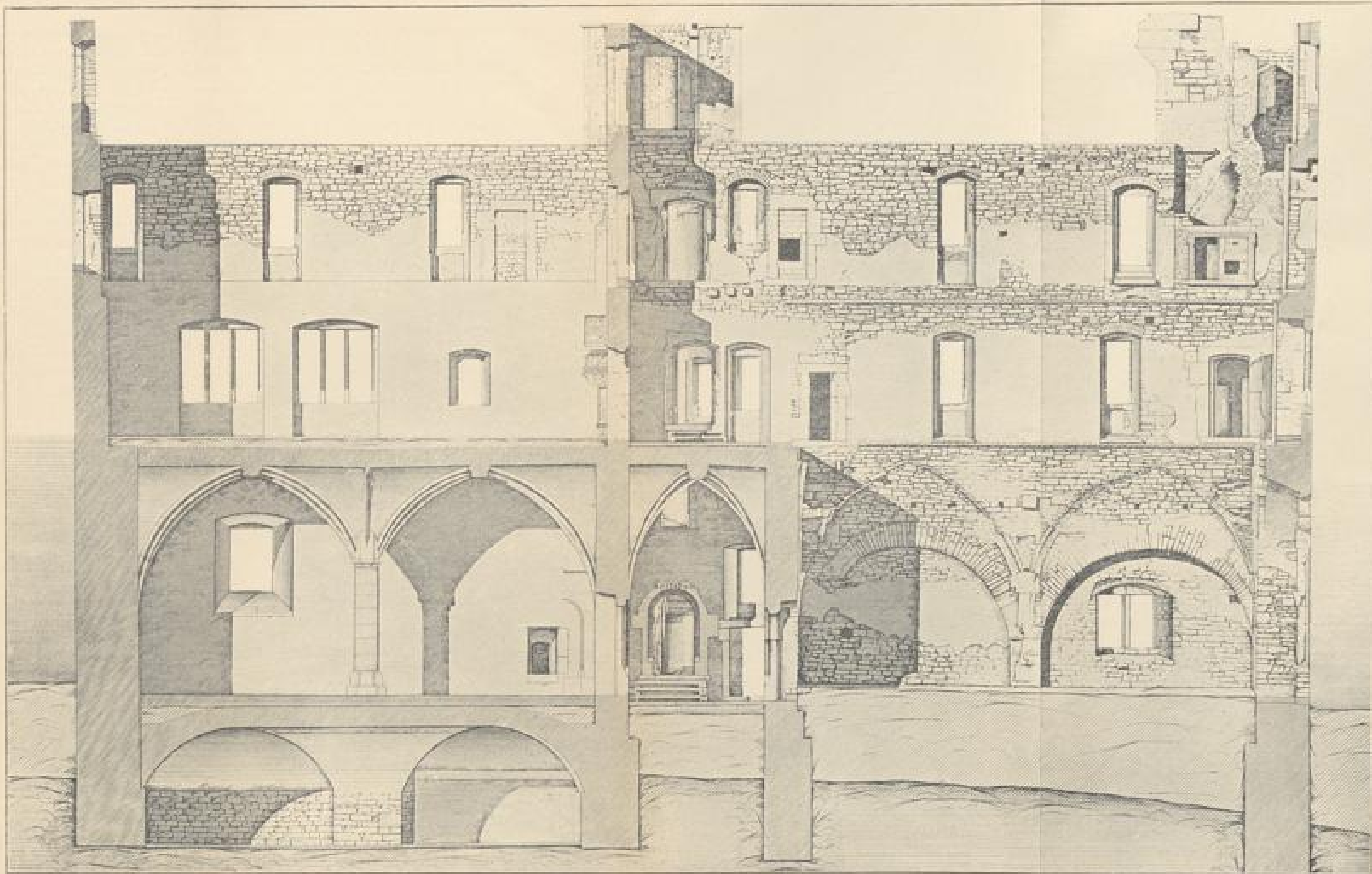
Fig. 273. Längsschnitt durch die Kapelle. (Nach Koch und Seitz.)
