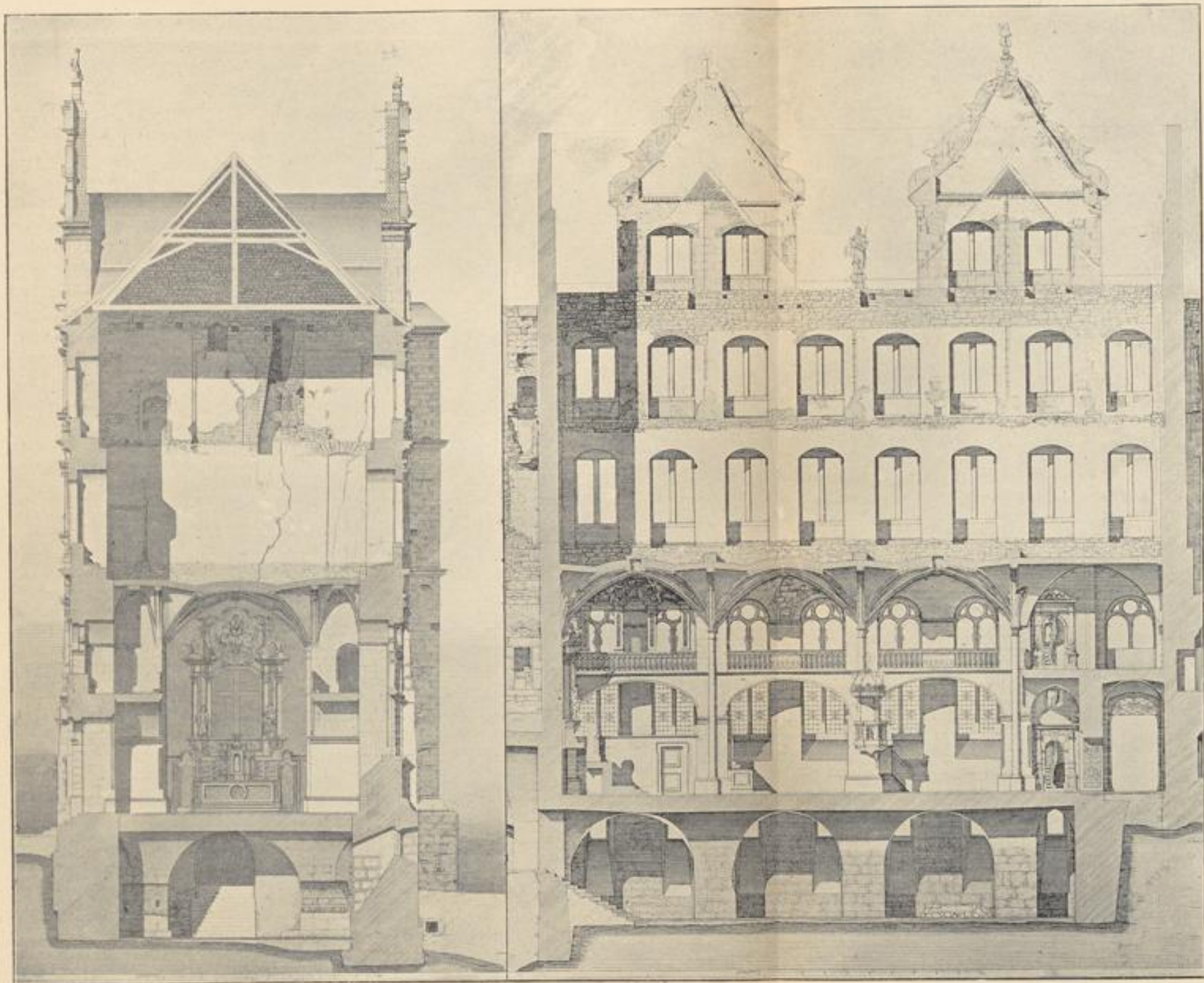
Fig. 318. Querschnitt und Längsschnitt des Friedrichsbaues. (Nach Koch und Seitz.)
