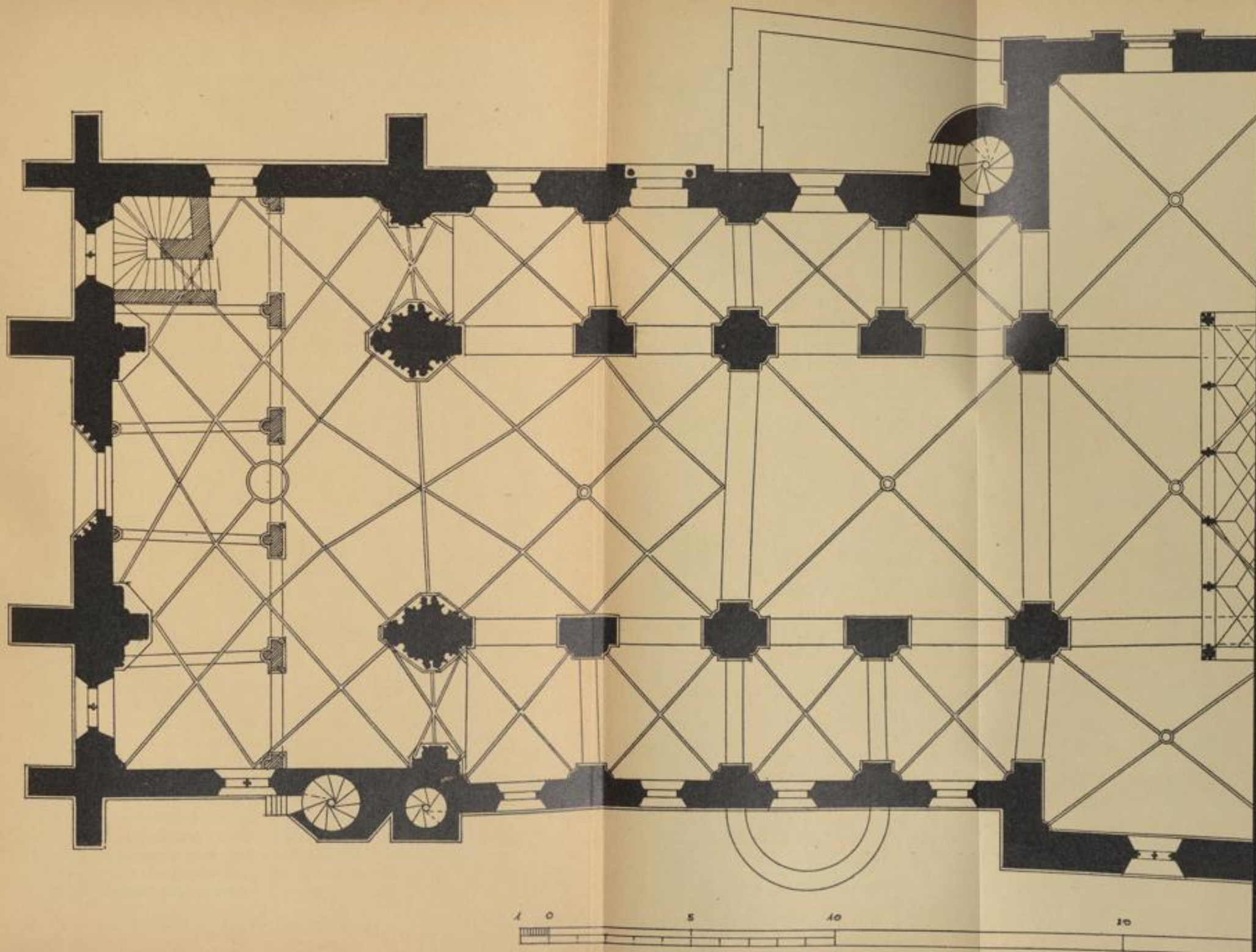
Fig. 12. Breisach. Grundriss des Münsters.
