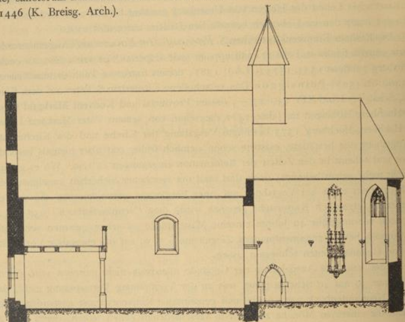
Längsschnitt.
