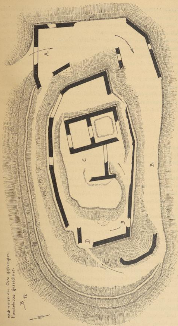
Fig. 115. Ruine Wiesneck. Grundriss.
