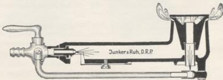
(Schnitt des Original-Junker & Ruh-Doppelsparbrenners, mehrfach patentiert)
