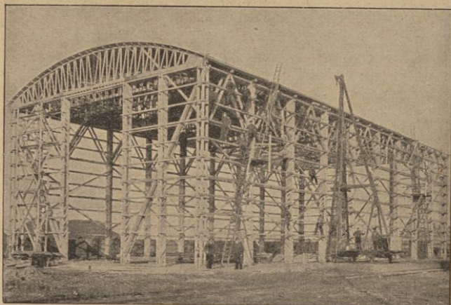
Lagerhalle gebaut mit Holzverbinder „BULLDOG“
